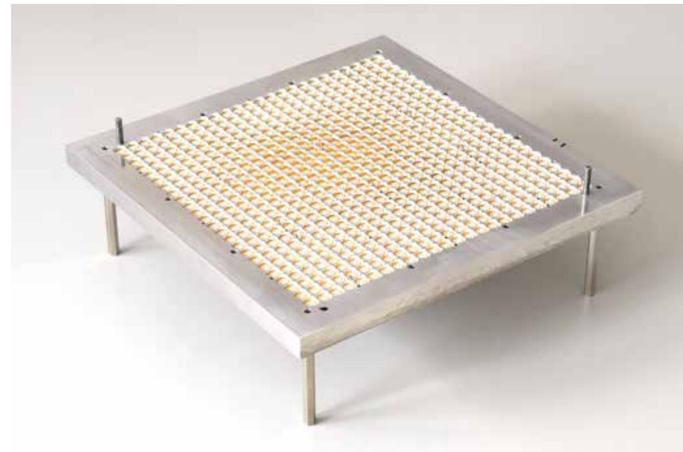
Abb. 2: Planarantenne für 30 GHz mit elektronischer Strahlschwenkung bestehend aus 9 Einzelmodulen mit je 64 Elementen in einem Metallrahmen
